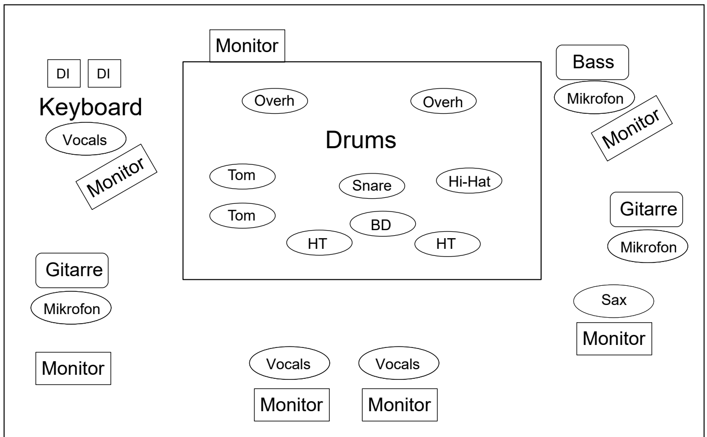
Bühnenplan
